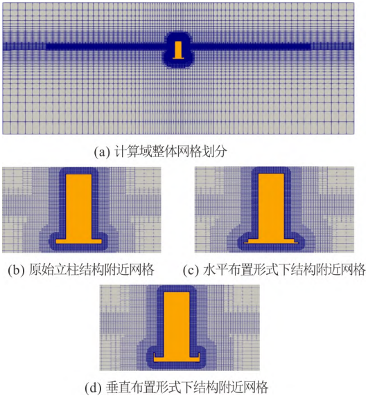
图4 网格划分
