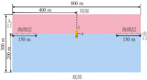
图3 计算域
