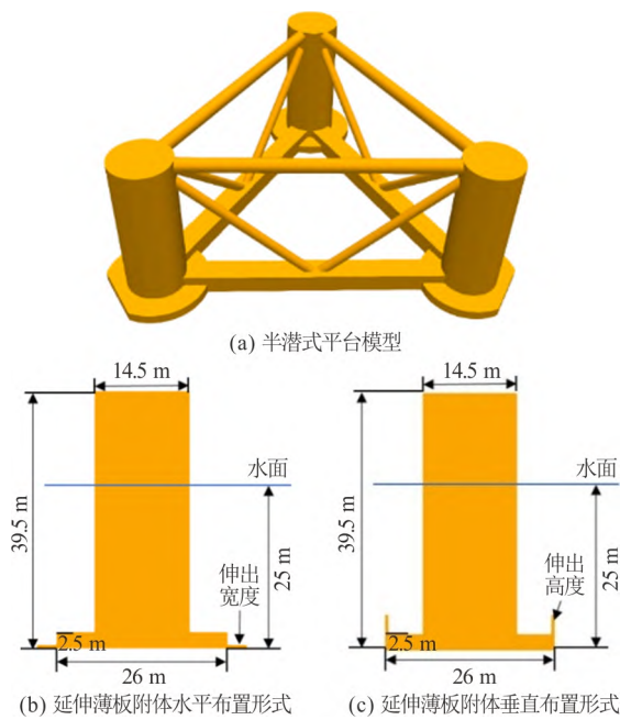
图2 模型结构样式与延伸薄板布置形式
