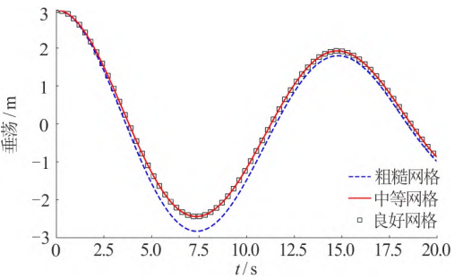
图5 网格收敛性分析
